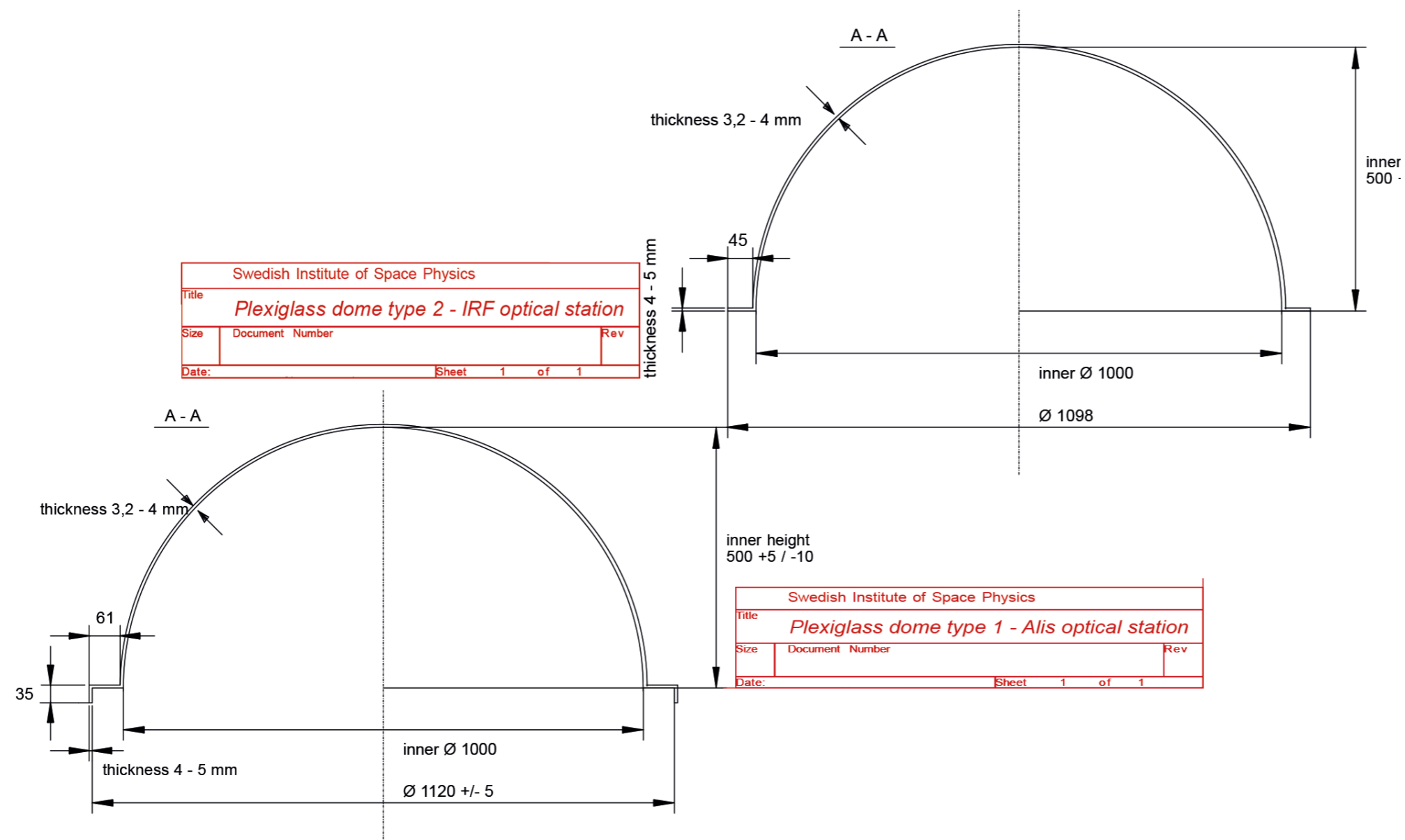
Bild 3.2: IRF:s optiska observatorieinstrument är monterade under plexiglasskupoler. Exempelvis firmamentkameran som tar bilder av himlavalvet och bland annat registrerar norrskenförekomst och molnighet.
