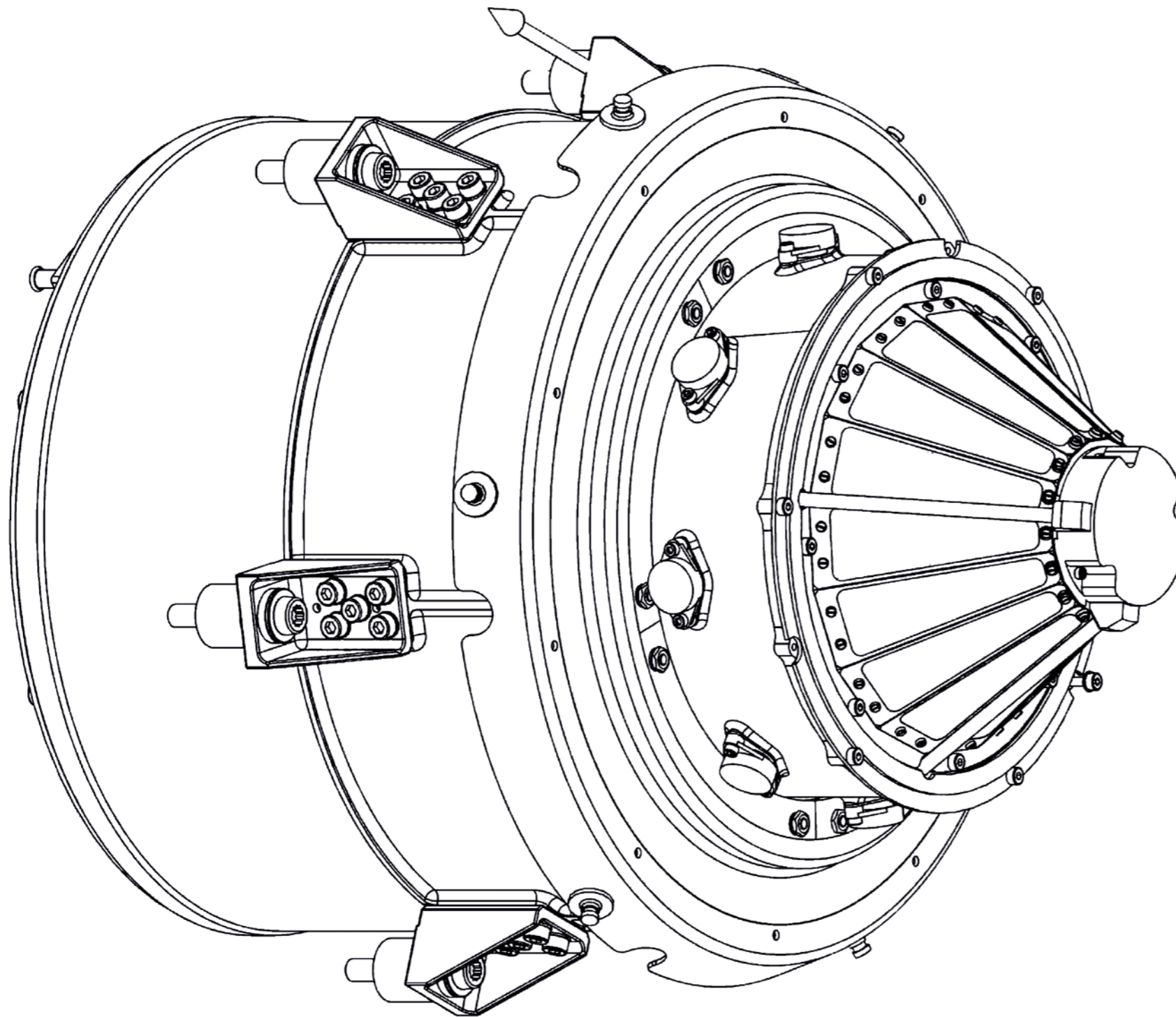
Bild 2.7: IRF-sensorn Jovian plasma Dynamics and Composition Analyzer (JDC) ska mäta joner och elektroner i Jupitersystemet och tillhör ett instrumentpaket med sex sensorer som leds av IRF.
