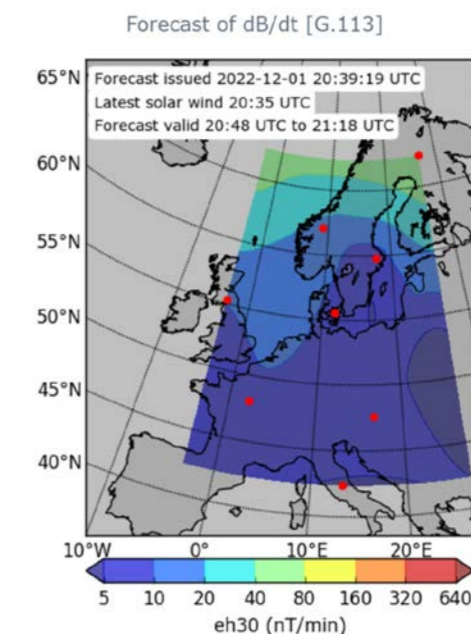
Bild 2.6: Exempel på prognos för variationer i jordens magnetfält över Europa den 1 december baserat på IRF:s dB/dT-2018-modellen i det europeiska projektet Space Weather Service Network (SWESNET) inom ESA och dess geomagnetiska expertservicecentrum G-ESC.
